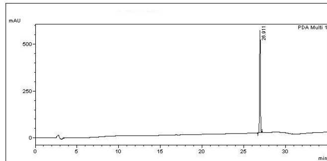
ภาพที่ 3 HPLC ของสารมาตรฐาน \alpha -Mangostin
