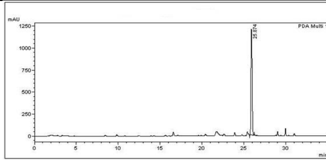
ภาพที่ 2 HPLC ของสารสกัดเปลือกมังคุด จ.ชุมพร
